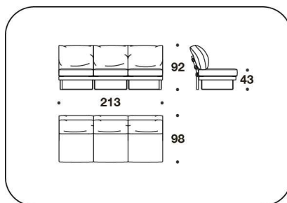
TOA (AE3CN) ELEMENTO SEDUTA 3 POSTI SENZA BRACCIOLI / 3 SEATER ELEMENT WITHOUT ARMS 213x98x92H. - H.S.43cm 84x38 2/3x36 1/3H. - H.S.17"
