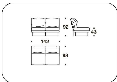
TOA (AE2CN) ELEMENTO SEDUTA 2 POSTO SENZA BRACCIOLI / 2 SEATER ELEMENT WITHOUT ARMS 142x98x92H. - H.S.43cm 56x38 2/3x36 1/3H. - H.S.17"
