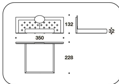
CME (KUSA) KING USA : LETTO PER MATERASSO / BED FOR MATTRESS 195x205 - 350x228x132H. - H.B.32cm 76 2/3x80 2/3 - 137 2/3x89 2/3x52H. - H.B.12 2/4"
