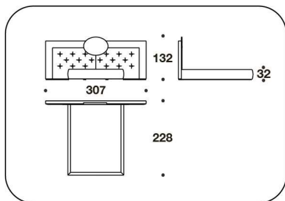
CME (QUSA) QUEEN USA : LETTO PER MATERASSO / BED FOR MATTRESS 152x205 - 307x228x132H. - H.B.32cm 60x80 2/3 - 121x89 2/3x52H. - H.B.12 2/4"
