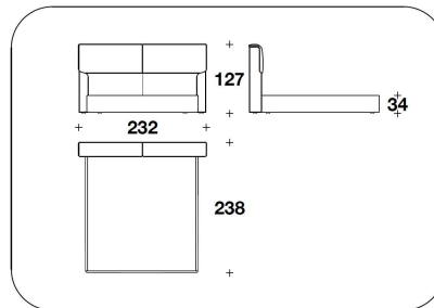
KIA (KUSA) KING USA : LETTO PER MATERASSO / BED FOR MATTRESS 195x205 - 232x238x127H. - H.B.34cm 76 2/3x80 2/3 - 91 1/3x93 2/3x50H. - H.B.13 2/4"
