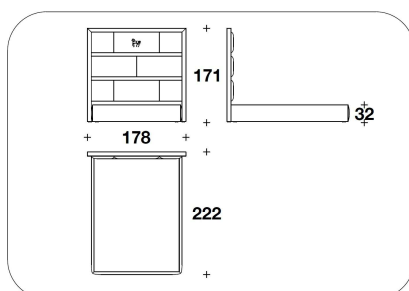
ZFR (QUSA) QUEEN USA : LETTO PER MATERASSO / BED FOR MATTRESS 152x205 - 178x222x171H. - H.B.32cm 60x80 2/3 - 70x87 1/3x67 1/3H. - H.B.12 2/4"
