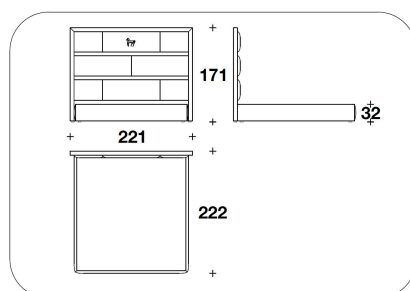
ZFR (KUSA) KING USA : LETTO PER MATERASSO / BED FOR MATTRESS 195x205 - 221x222x171H. - H.B.32cm 76 2/3x80 2/3 - 87x87 1/3x67 1/3H. - H.B.12 2/4"
