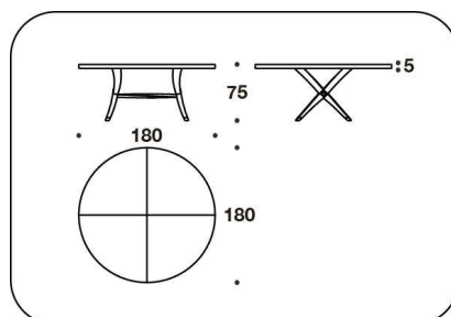
TAV (T63P) - TAV (T63E) - TAV (T63R) - TAV (T63RA)
