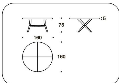
TAV (T65P) - TAV (T65E) - TAV (T65R) - TAV (T65RA)
