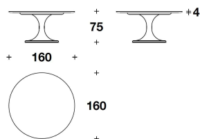
TTV (16LP) TAVOLO / TABLE Ø 160x75H. - THK.4cm Ø 63x29 2/3H. - THK.1 9/16"
